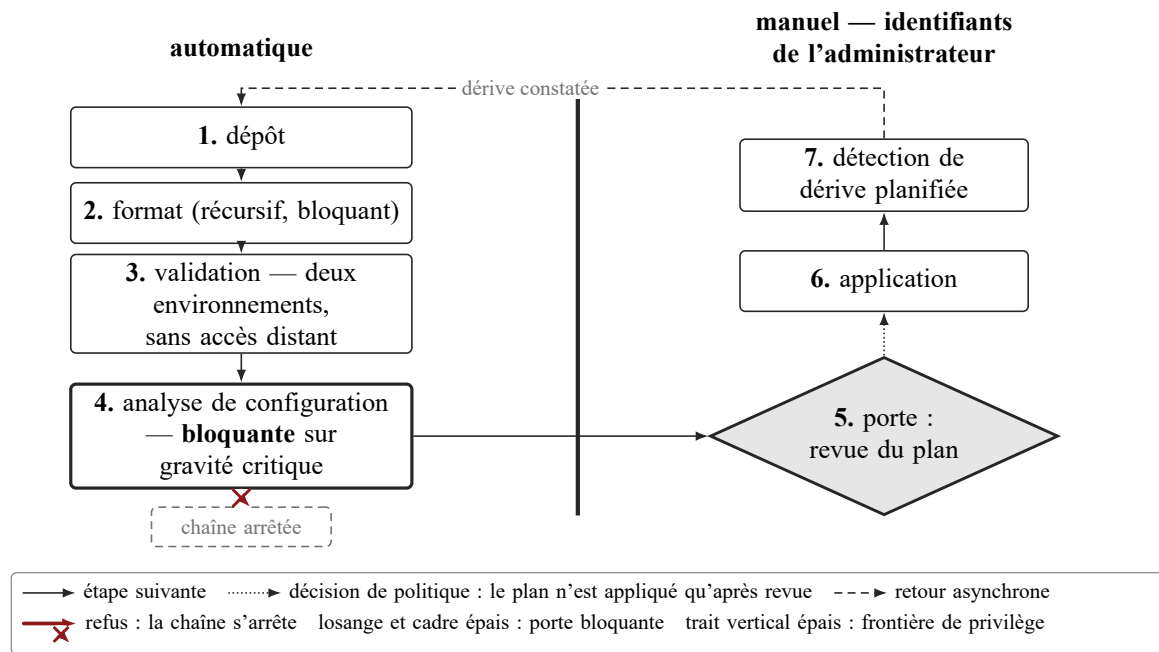
FIG. 20. Chaîne de provisionnement de l'infrastructure : la frontière automatique/manuel est un choix de privilège , non un degré d'achèvement — la partie automatisée n'a, par construction, aucun accès au fournisseur cloud.
